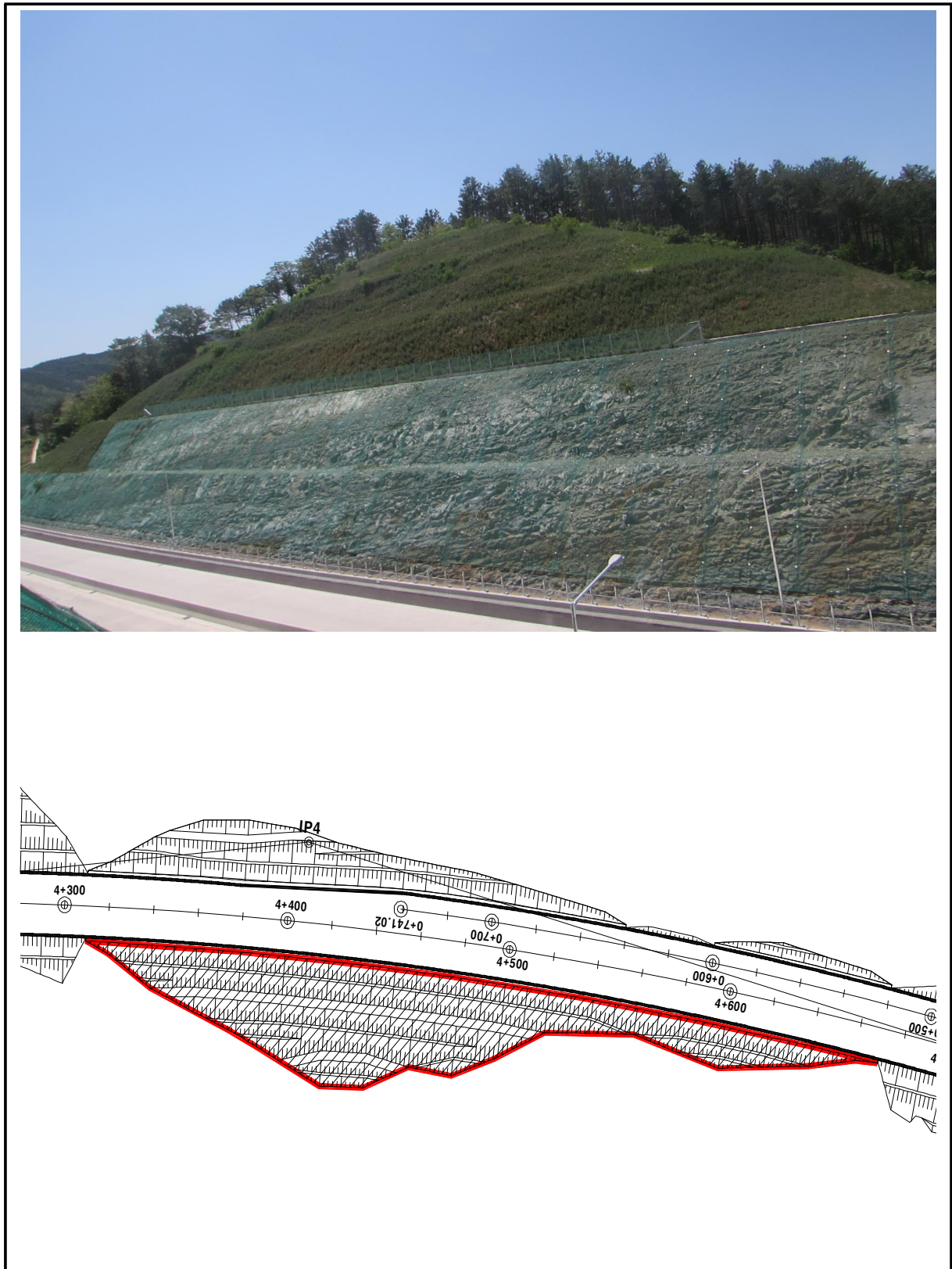
【그림 32.14】 영천절토32 검토대상 비탈면구간
