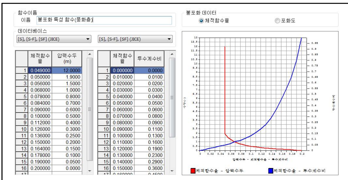
<그림 32-15> 압력수두-체적함수물(포화도)-투수계수비 함수
