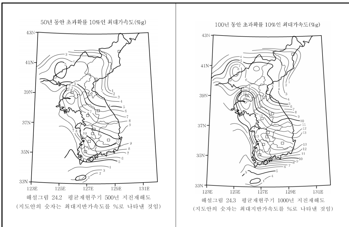
【그림 32.12】 평균재현주기 500년 및 1000년 지진재해도
